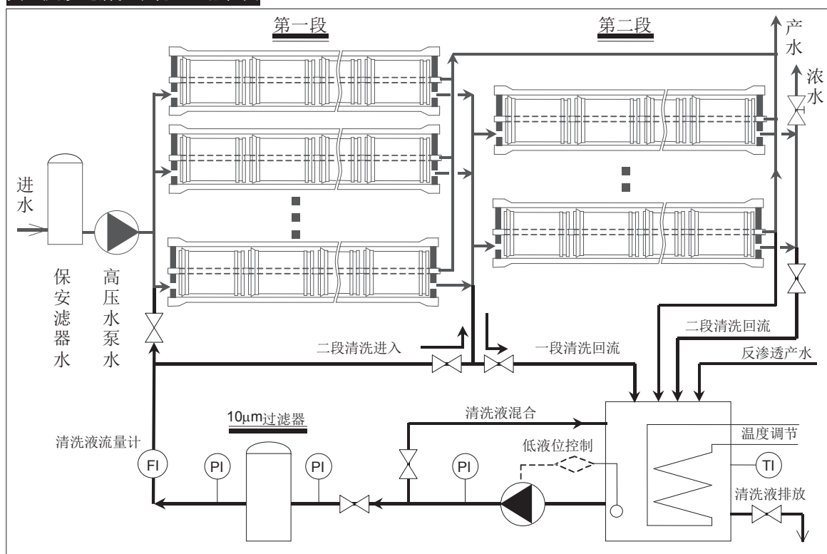
典型反渗透清洗系统工艺流程图
