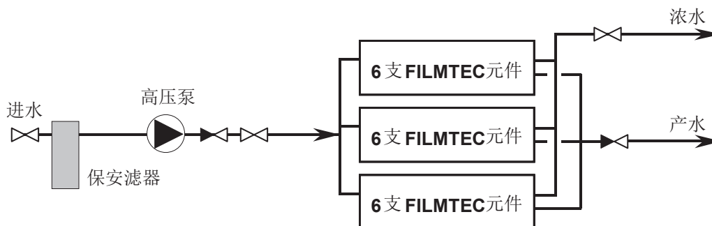
图 5-4 单段系统
