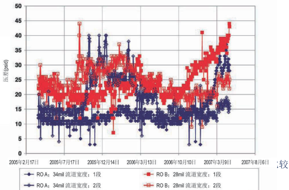
图 1. 34mil 流道宽度和 28mil 流道宽度的元件的压差比较
