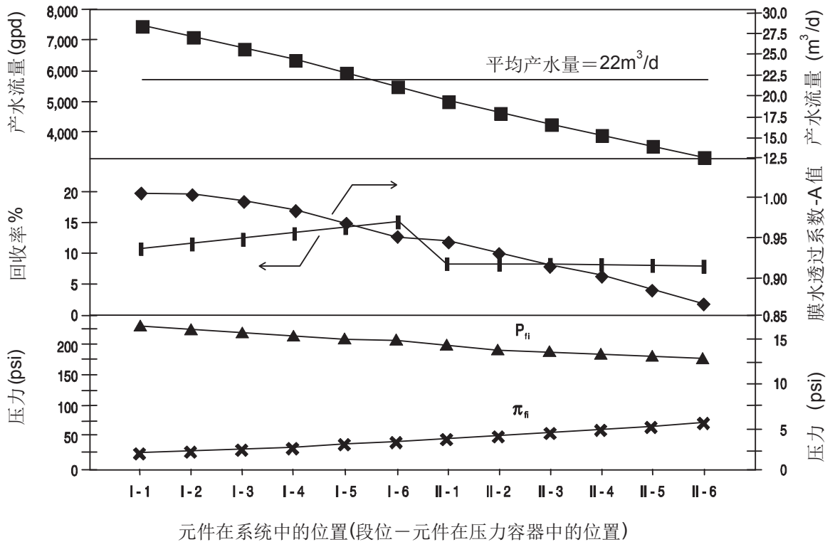
图 5-11 8 英寸 BW30 元件在 2:1 排列系统中每支元件性能变化趋势
