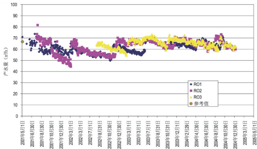
图 1：产水流量性能（按照设计启动性能进行标准化）
