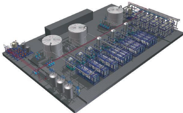
UF + RO + MB系统3D效果图
