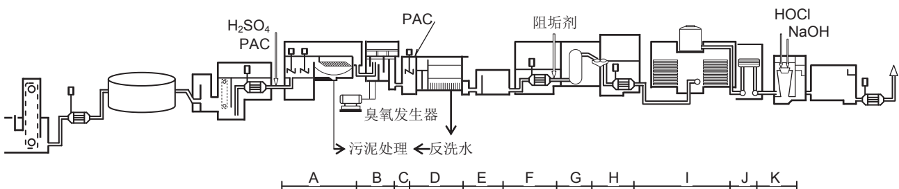
图 1. 膜法水处理系统, 第 2 系列
