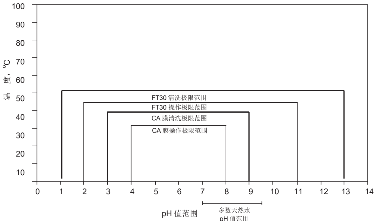
图 3. FILMTEC™ FT30 超薄复合膜和 CA 膜运行和清洗参数比较
