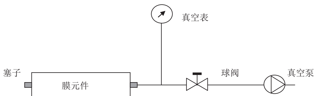
图 1. 真空度下降速率试验
