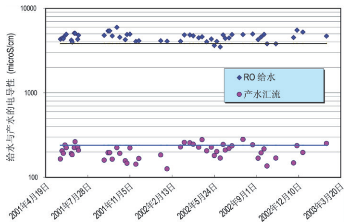
图 2：2001 年 4 月到 2003 年 3 月间反渗透给水和来自各装置的产水汇流的电导率
