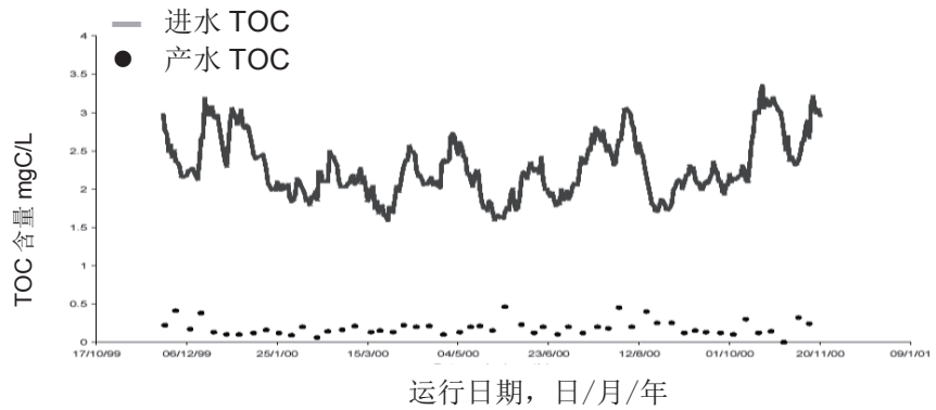
图 12 进水和产水 TOC 含量 (mgC/L)
