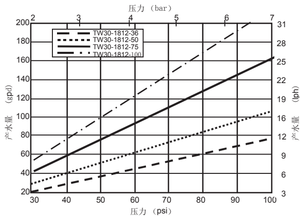
压力对产水量的影响 (恒定温度和回收率)
