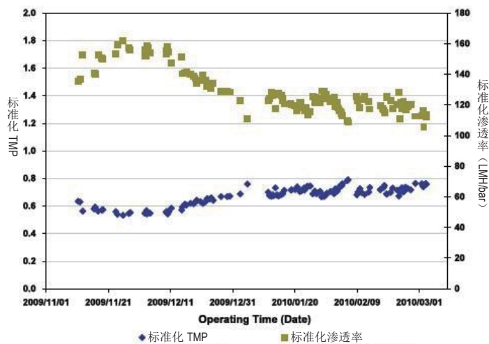
图 5. 超滤系统性能：标准化 TMP 以及标准化渗透率
