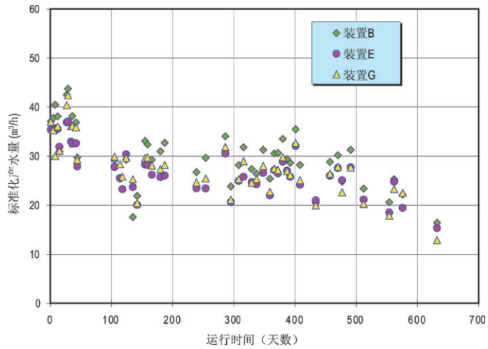
图 5: 采用新膜元件的三套 RO 装置的标准化流量
