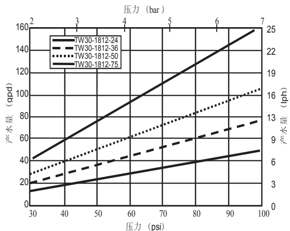
图 2. 压力对产水量的影响 (固定温度和回收率)
