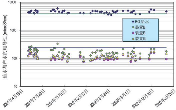
图 4: 采用新膜元件的三套 RO 装置的平均除盐率数据
