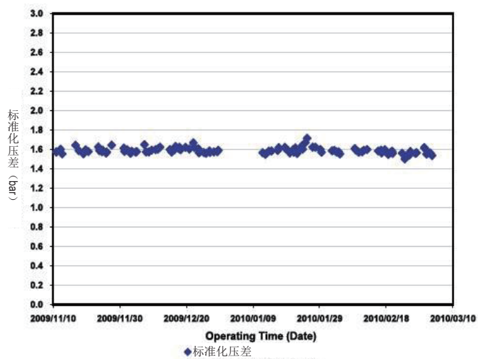
图 7. 反渗透系统性能：三段系统标准化压差
