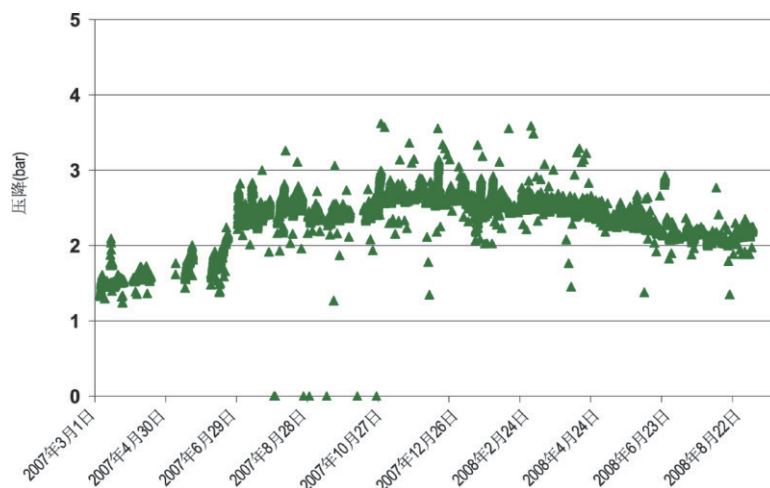
图 4. 一级RO压降（进水至浓水）
