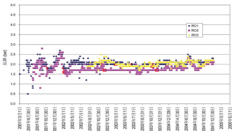
图 3: 从进水到浓水的系统压差
