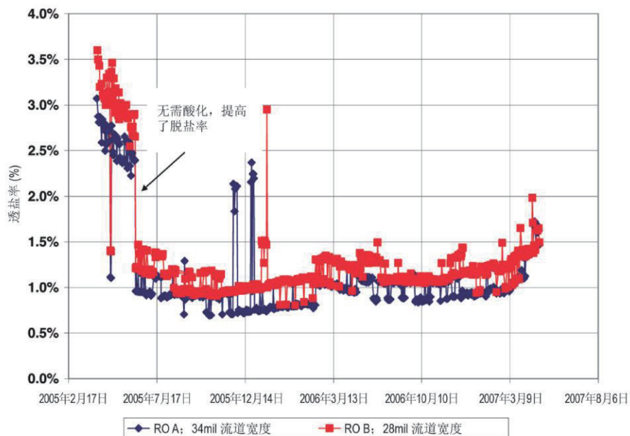
图 3. 34mil 流道宽度和 28mil 流道宽度的元件的透盐率比较
