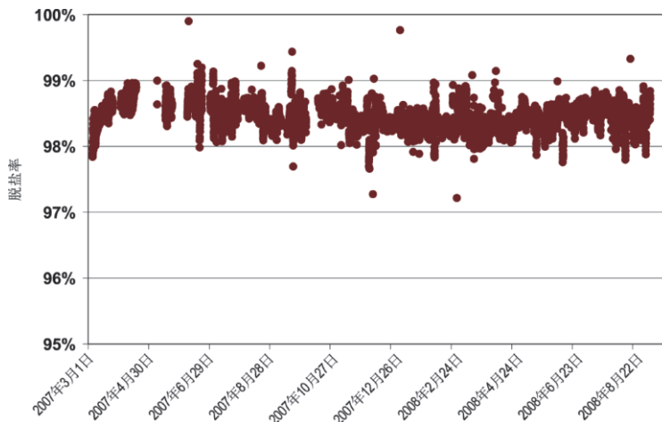
图 3. 一级RO标准脱盐率
