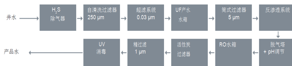
图 3. 工厂工艺流程图
