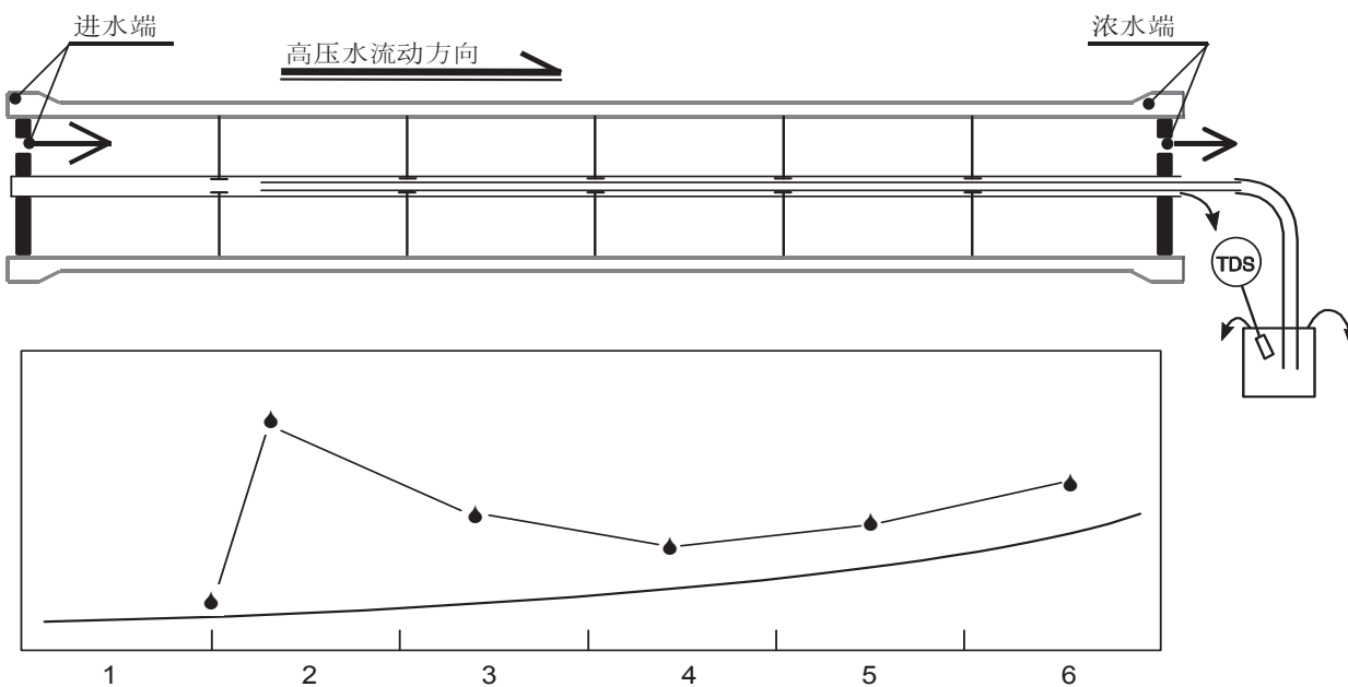
图 9-2 产水电导率分布规律
