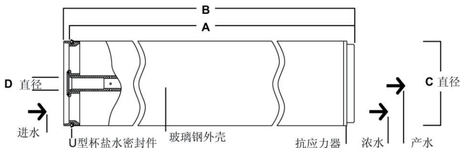
外形尺寸 - 英寸 (mm)
