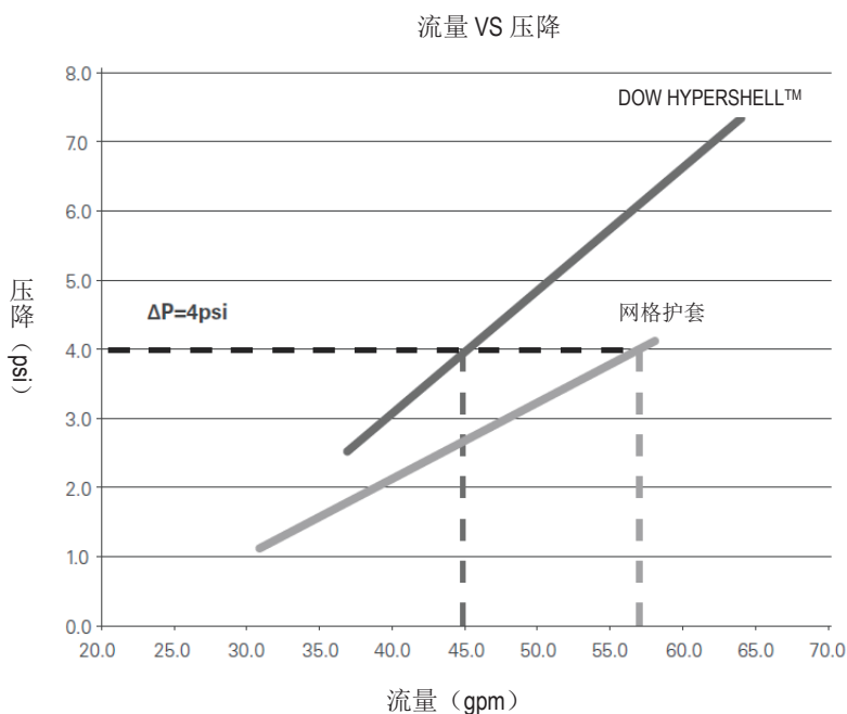
图 1，普通网格护套和 HYPER SHELL 8038 膜元件进水流量压降对比。HYPER SHELL™ 具有更小的外壳旁流量，在同等压降下，相对普通网格护套膜元件，其进水流量降低约 30%。图 1 说明在 4psi 压降下的流量对比，通过降低流量可以降低系统能耗。
