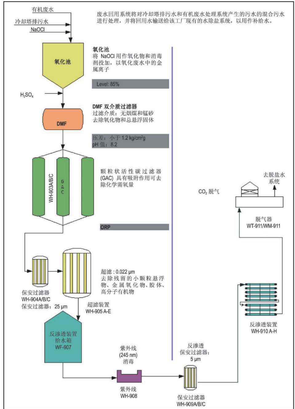
图 1. 最终工艺流程图
