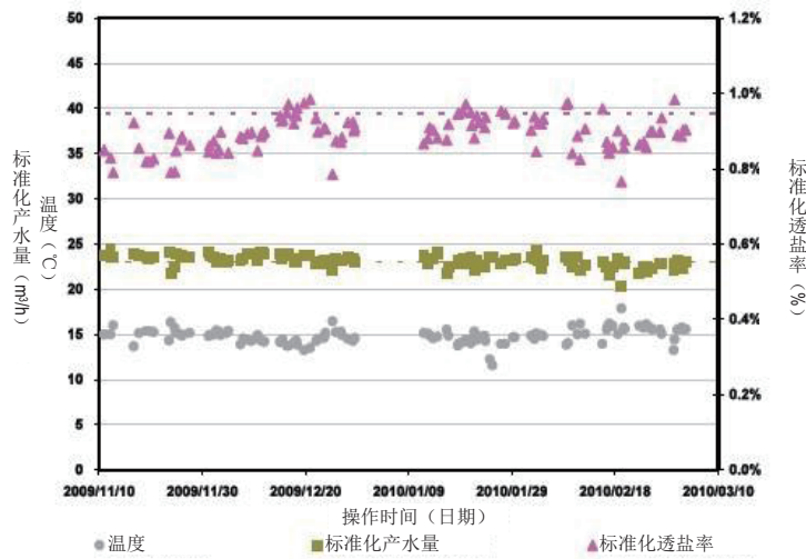
图 6. 反渗透系统性能：标准化渗透率及透盐率
