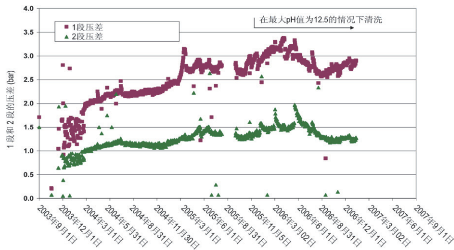
图 3：4#RO 装置每段的压差
