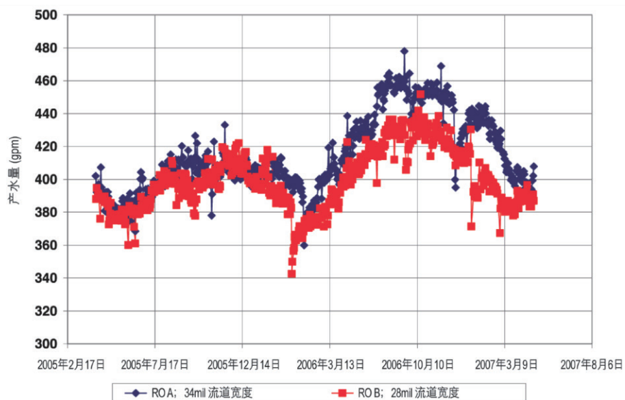
图 1. 34mil 流道宽度和 28mil 流道宽度的元件的标准化产水量比较
