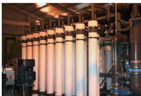
UF 系统
