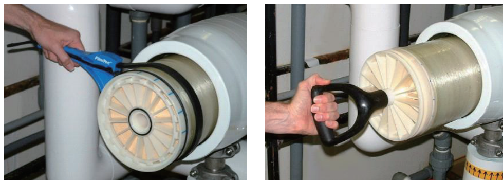
图 2. 用于端面自锁膜元件安装的轻型带钳（左）和拉手（右）
