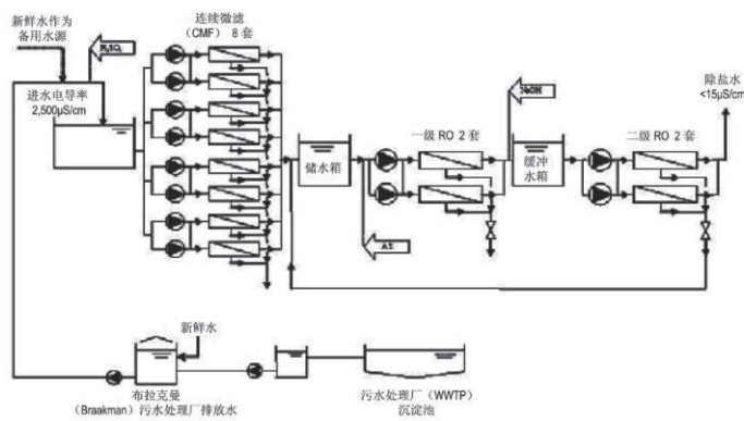
图 1. 改造后的全膜系统的工艺流程图
