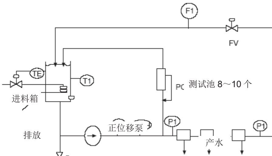
图 1. 膜片测试池和元件测试装置
