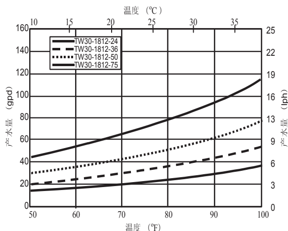
图 3. 温度对产水流量的影响 (固定压力和回收率)
