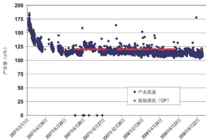
图 2. 一级RO标准产水流量以及就地清洗CIP事项
